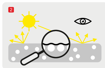
Rys. 2 Dodatek koncentratu matującego, światło rozprasza się równomiernie na kontrolowanych nierównościach powierzchni (efekt matowy)
